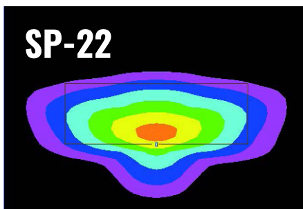
Energiatehokas optiikka erittäin pitkällä pylväsvälillä. Antaa tasaista valoa myös märissä olosuhteissa. Sopii myös kevyen liikenteen väylille/pururadoille.
