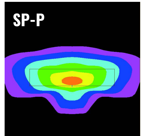
Tasainen yleisvalo-optiikka esimerkiksi teiden kaksipuoliseen reunavalaistukseen tai rampeihin. Sopii erittäin pitkälle pylväsvälille. Toimii parhaiten etäällä tiestä.
