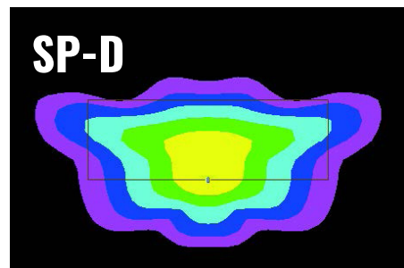
Leveälle tielle ja pitkälle pylväsvälille sopiva optiikka. Antaa paljon takavaloa.
