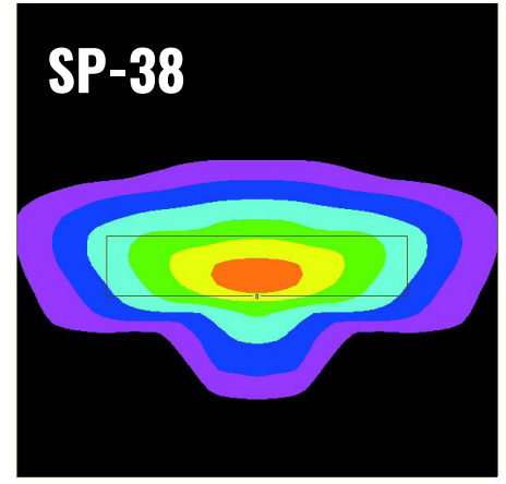
Keskikaistalle asennettava moottoritieoptiikka. Sopii erityisesti korkeisiin pylväisiin ja erityisen pitkille, jopa 100 metrin pylväsväleille.
