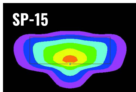
Yleisvalaisin teille erittäin pitkällä pylväsvälillä. Antaa tasaista valoa myös märissä olosuhteissa. Leveähkö tieprofiili (valaisee myös vastakkaisen kevyen liikenteen väylän jos pylväsväli on lyhyempi).
