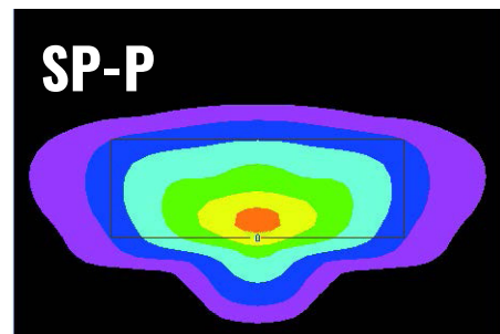
Yleisoptiikka tonttikaduille erittäin pitkällä pylväsvälillä. Antaa tasaista valoa myös märissä olosuhteissa, kun pylväk on etäällä tiestä. Sopii myös melko leveille teille ja kevyen liikenteen väylille/pururadoille.
