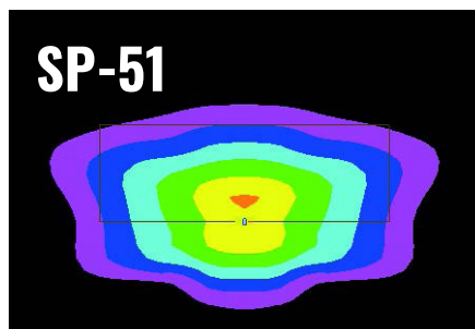
Optiikka, joka antaa runsaasti takavaloa. Pitkälle pylväsvälille. Erityisen energiatehokas, jos kevyen liikenteen väylä on sijoitettu pylvään taakse.
